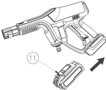
Presione los botones y extraiga la batería
